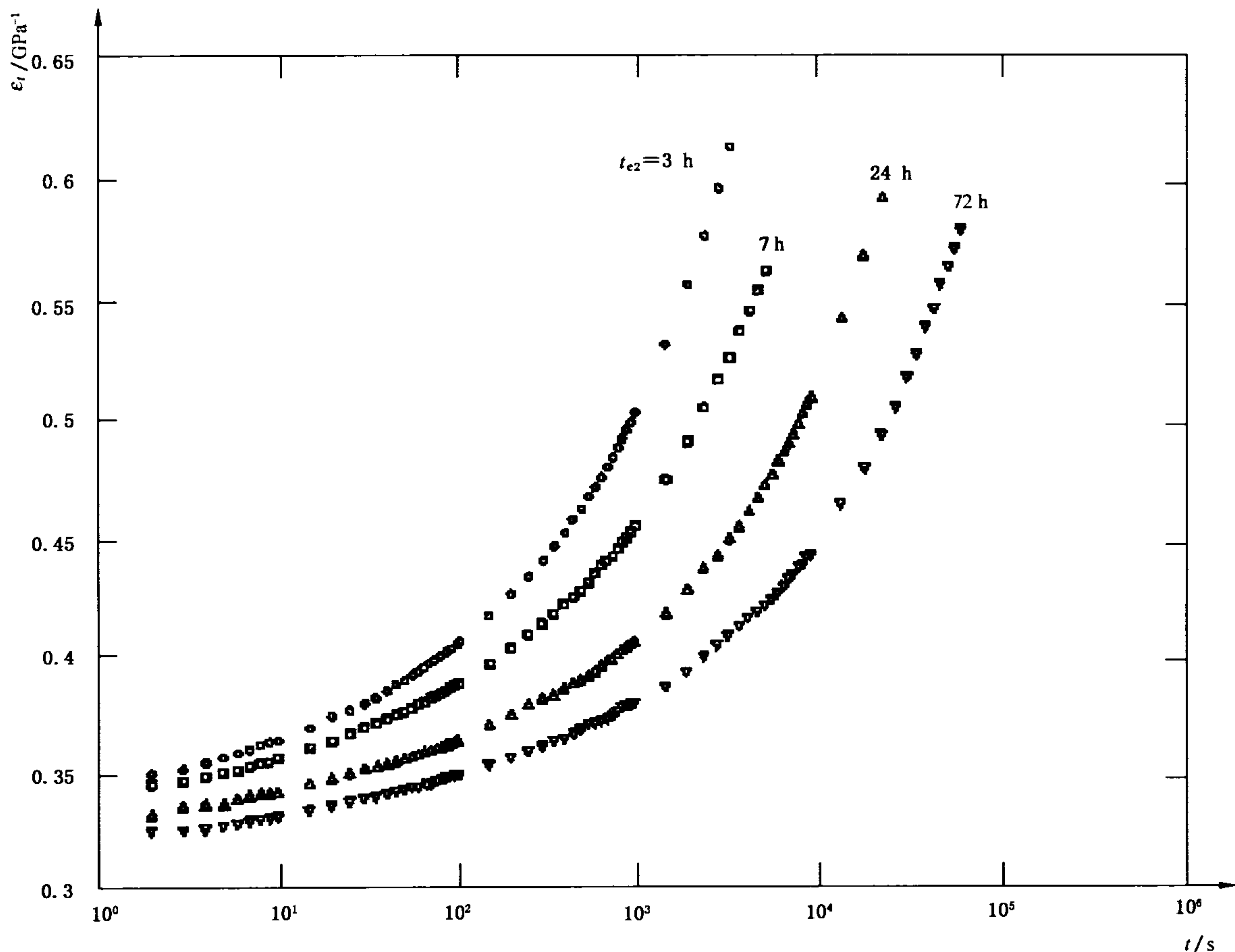
图 A.2 由 23 °C 加热至 44 °C 并保温不同时间 t_2 的 PVC 试样蠕变曲线 (试样加热前已在 23 °C 下存放 200 h)
