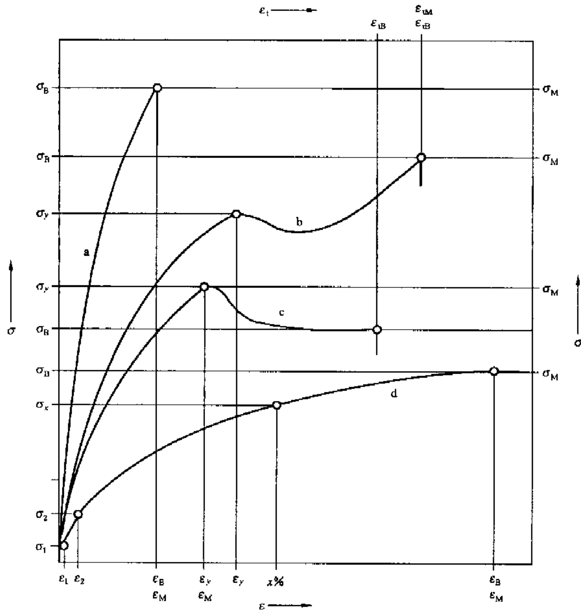
曲线 a 脆性材料 曲线 b 和 c 有屈服点的韧性材料 曲线 d 无屈服点的韧性材料
